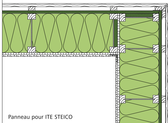
W2 Angle de mur extérieur avec STEICOjoist
